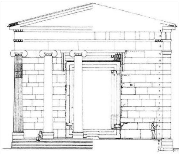
Αριστερά: Αρχιτεκτονικά μέλη του ναού της Αθηνάς στο Κάστρο Δεξιά: Γραφική αποκατάσταση της πρόσοψης του ναού
